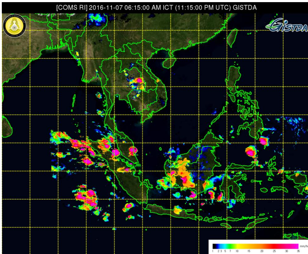
ภาพที่ 1 ข้อมูลจากดาวเทียม COMS แสดงสภาพอากาศ ณ วันที่ 7 พฤศจิกายน 2559 เวลา 06.15 น.
