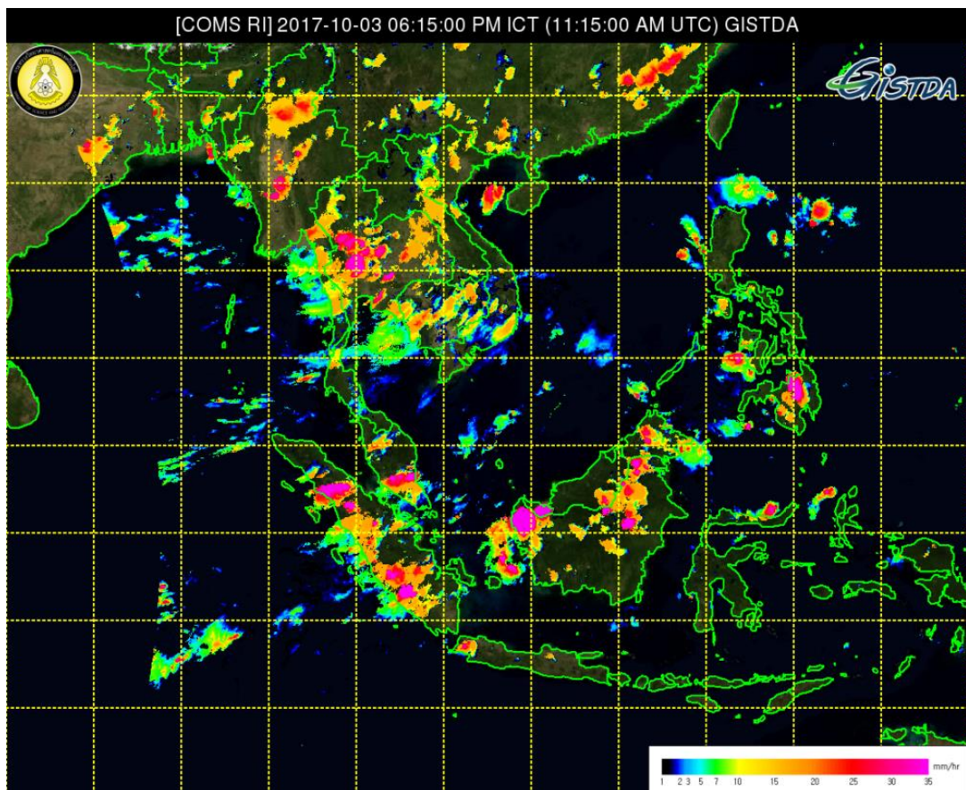
ภาพที่ 1 ข้อมูลจากดาวเทียม COMS แสดงสภาพอากาศ ณ วันที่ 3 ตุลาคม 2560 เวลา 18.15 น
