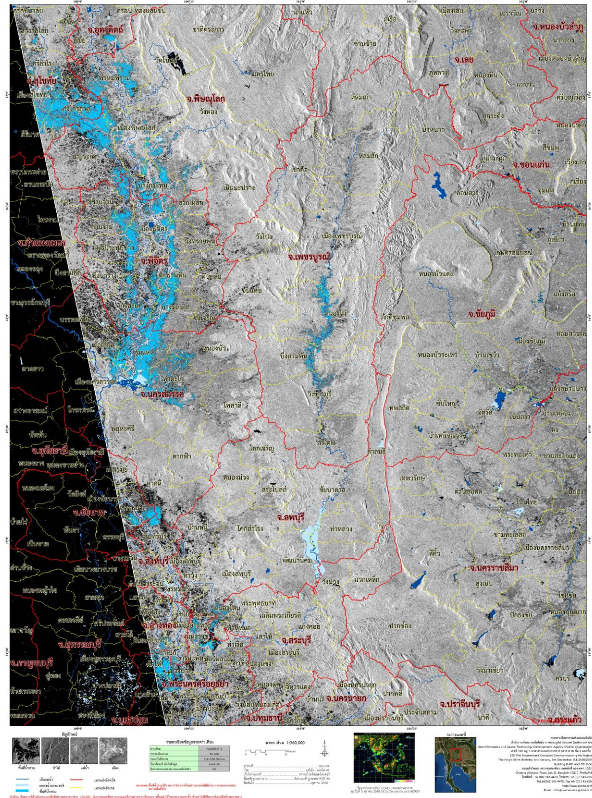
ภาพที่ 1 พื้นที่น้ำท่วม (สีฟ้า) จากการวิเคราะห์ข้อมูลจากดาวเทียม บันทึกภาพ Radarsat-2 วันที่ 3 ตุลาคม 2560 เวลา 18.24 น. บริเวณบางส่วนของจังหวัดพิจิตร พิษณุโลก นครสวรรค์ สุโขทัย พระนครศรีอยุธยา เพชรบูรณ์ ชัยนาท อ่างทอง สิงห์บุรี สระบุรี อุตรดิตถ์ และลพบุรี
