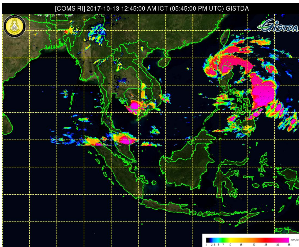
ภาพที่ 1 ข้อมูลจากดาวเทียม COMS แสดงสภาพอากาศ ณ วันที่ 12 ตุลาคม 2560 เวลา 17.45น.
