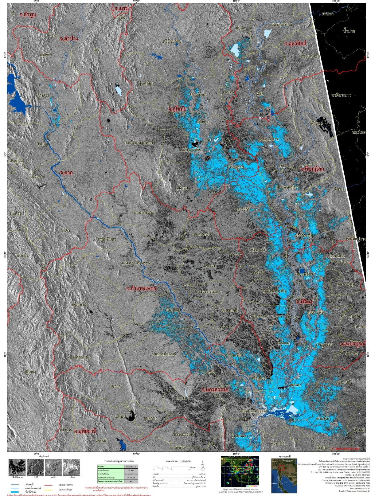
ภาพที่ 2 พื้นที่น้ำท่วม (สีฟ้า) จากการวิเคราะห์ข้อมูลจากดาวเทียม บันทึกภาพ Radarsat-2 วันที่ 13 ตุลาคม 2560 เวลา 18.33 น. บริเวณบางส่วนของจังหวัดนครสวรรค์ พิจิตร พิษณุโลก สุโขทัย กำแพงเพชร อุตรดิตถ์ พะเยา และตาก
