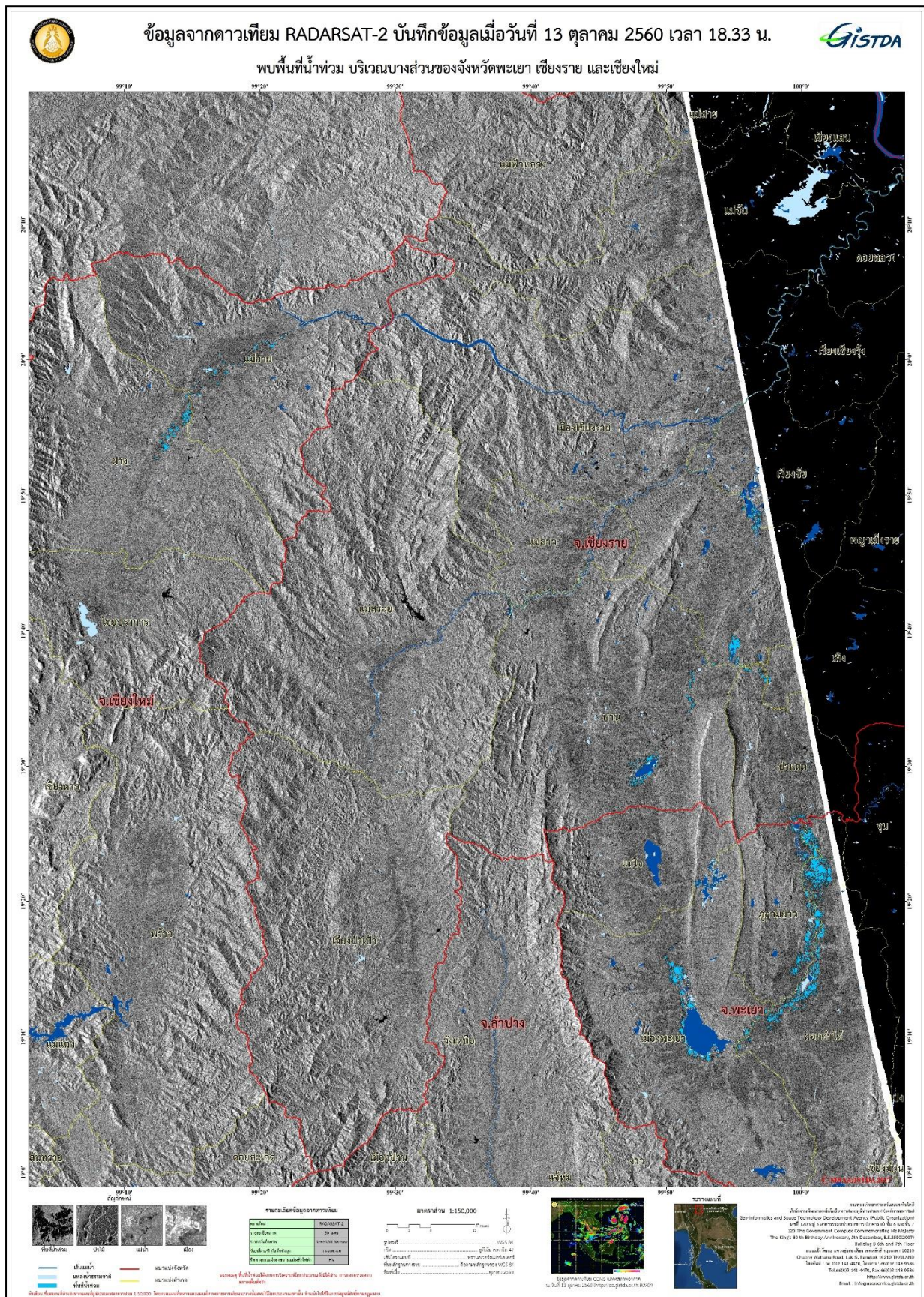
ภาพที่ 1 พื้นที่น้ำท่วม (สีฟ้า) จากการวิเคราะห์ข้อมูลจากดาวเทียม บันทึกภาพ Radarsat-2 วันที่ 13 ตุลาคม 2560 เวลา 18.33 น. บริเวณบางส่วนของจังหวัดพะเยา เชียงราย และเชียงใหม่
