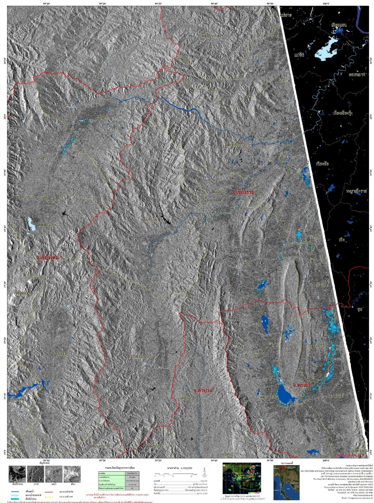
ภาพที่ 1 พื้นที่น้ำท่วม (สีฟ้า) จากดาวเทียม RADARSAT-2 บันทึกภาพ Radarsat-2 วันที่ 17 ตุลาคม 2560 เวลา 18.17 น. บริเวณบางส่วนของภาคตะวันออกเฉียงเหนือ
