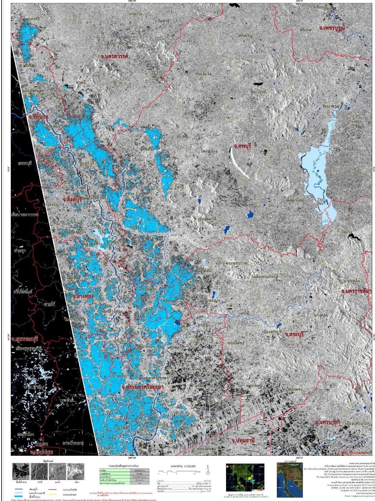
ภาพที่ 2 พื้นที่น้ำท่วม (สีฟ้า) จากการวิเคราะห์ข้อมูลจากดาวเทียม บันทึกภาพ Radarsat-2 วันที่ 27 ตุลาคม 2560 เวลา 18.24 น. บริเวณบางส่วนของจังหวัดนครสวรรค์ พระนครศรีอยุธยา ลพบุรี อ่างทอง สิงห์บุรี ชัยนาท และสระบุรี
