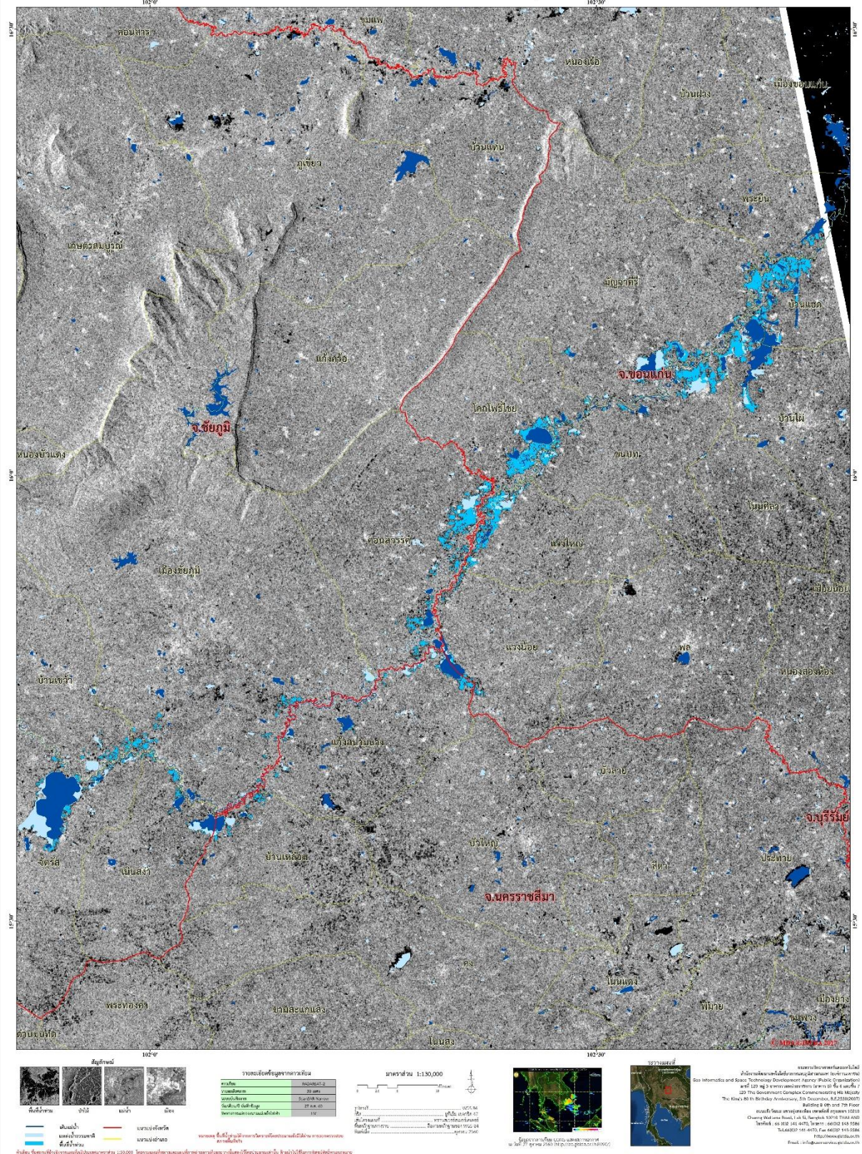
ภาพที่ 3 พื้นที่น้ำท่วม (สีฟ้า) จากการวิเคราะห์ข้อมูลจากดาวเทียม บันทึกภาพ Radarsat-2 วันที่ 27 ตุลาคม 2560 เวลา 18.24 น. บริเวณบางส่วนของจังหวัดขอนแก่น ชัยภูมิ และนครราชสีมา
