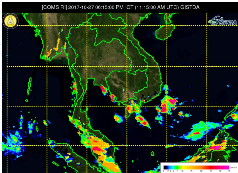
ภาพที่ 1 ข้อมูลจากดาวเทียม COMS แสดงสภาพอากาศ ณ วันที่ 27 ตุลาคม 2560 เวลา 18.15 น.
