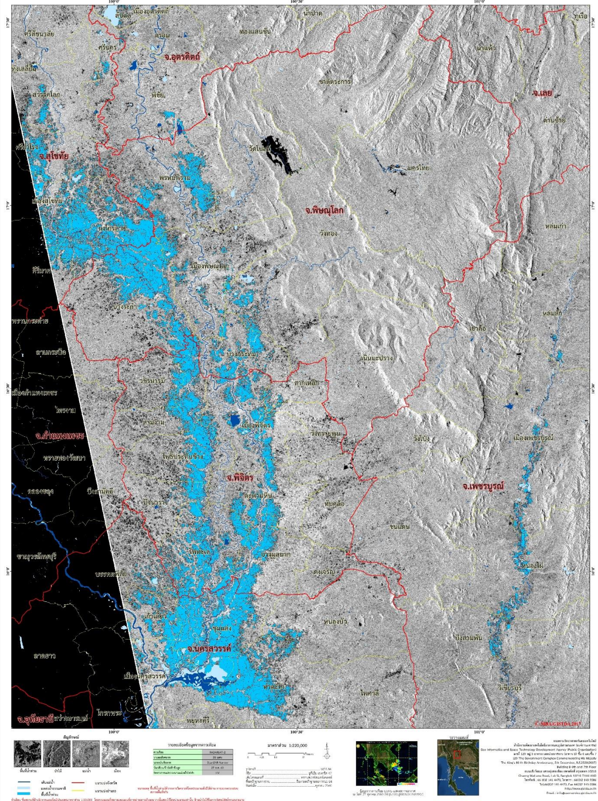
ภาพที่ 1 พื้นที่น้ำท่วม (สีฟ้า) จากการวิเคราะห์ข้อมูลจากดาวเทียม บันทึกภาพ Radarsat-2 วันที่ 27 ตุลาคม 2560 เวลา 18.24 น. บริเวณบางส่วนของจังหวัดนครสวรรค์ พิจิตร พิษณุโลก สุโขทัย เพชรบูรณ์ และอุตรดิตถ์
