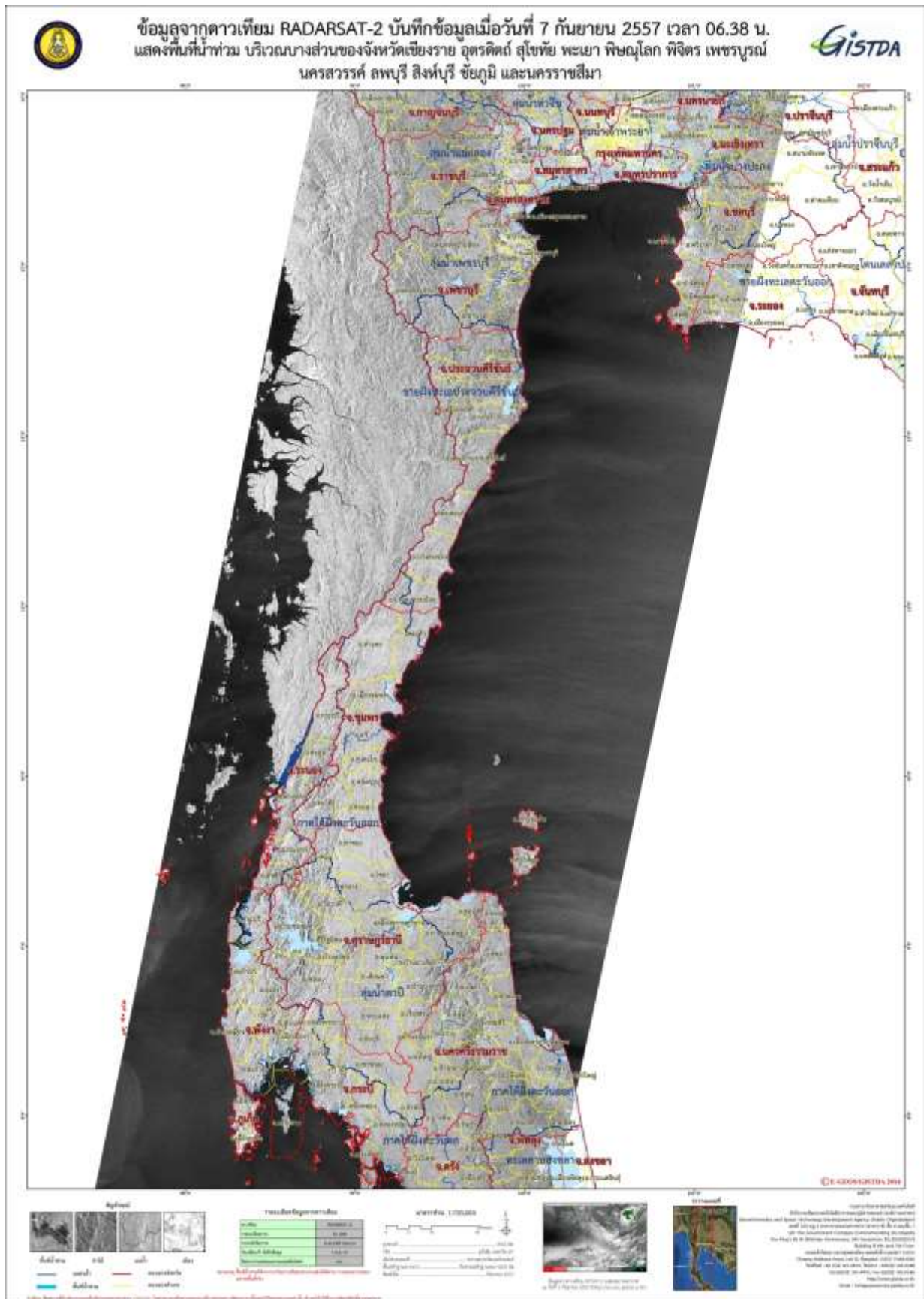
ภาพที่ 3 พื้นที่น้ำท่วม (สีฟ้า) จากการวิเคราะห์ข้อมูลจากดาวเทียม RADARSAT-2 บันทึกภาพวันที่ 7 กันยายน 2557 เวลา 06.38 น.บริเวณบางส่วนของจังหวัดเชียงราย อุตรดิตถ์ สุโขทัย พะเยา พิษณุโลก พิจิตร เพชรบูรณ์ นครสวรรค์ ลพบุรี สิงห์บุรี ชัยภูมิ และนครราชสีมา
