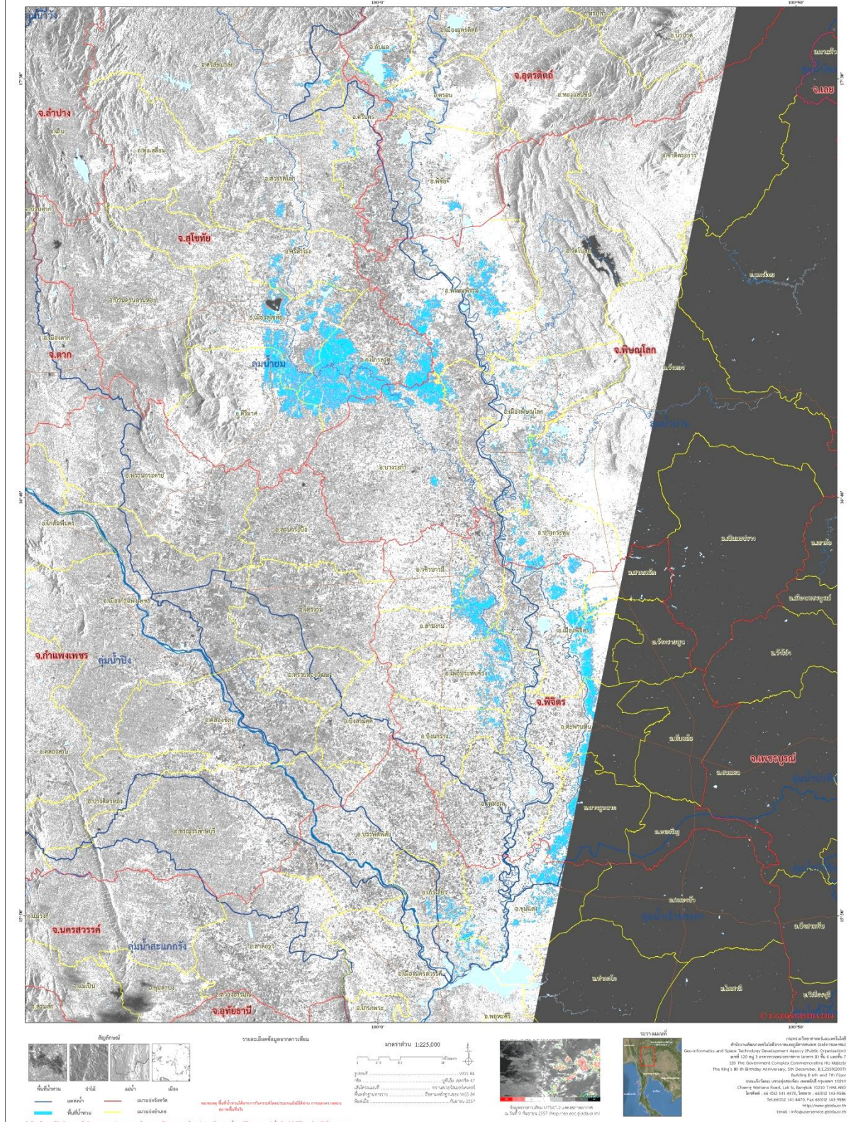
ภาพที่ 3 พื้นที่น้ำท่วม (สีฟ้า) จากการวิเคราะห์ข้อมูลจากดาวเทียม COSMO-SkyMed-2 บันทึกภาพเมื่อวันที่ 9 กันยายน 2557 เวลา 18.02 น. บริเวณบางส่วนของจังหวัดสุโขทัย พิจิตร พิษณุโลก นครสวรรค์ และอุตรดิตถ์
