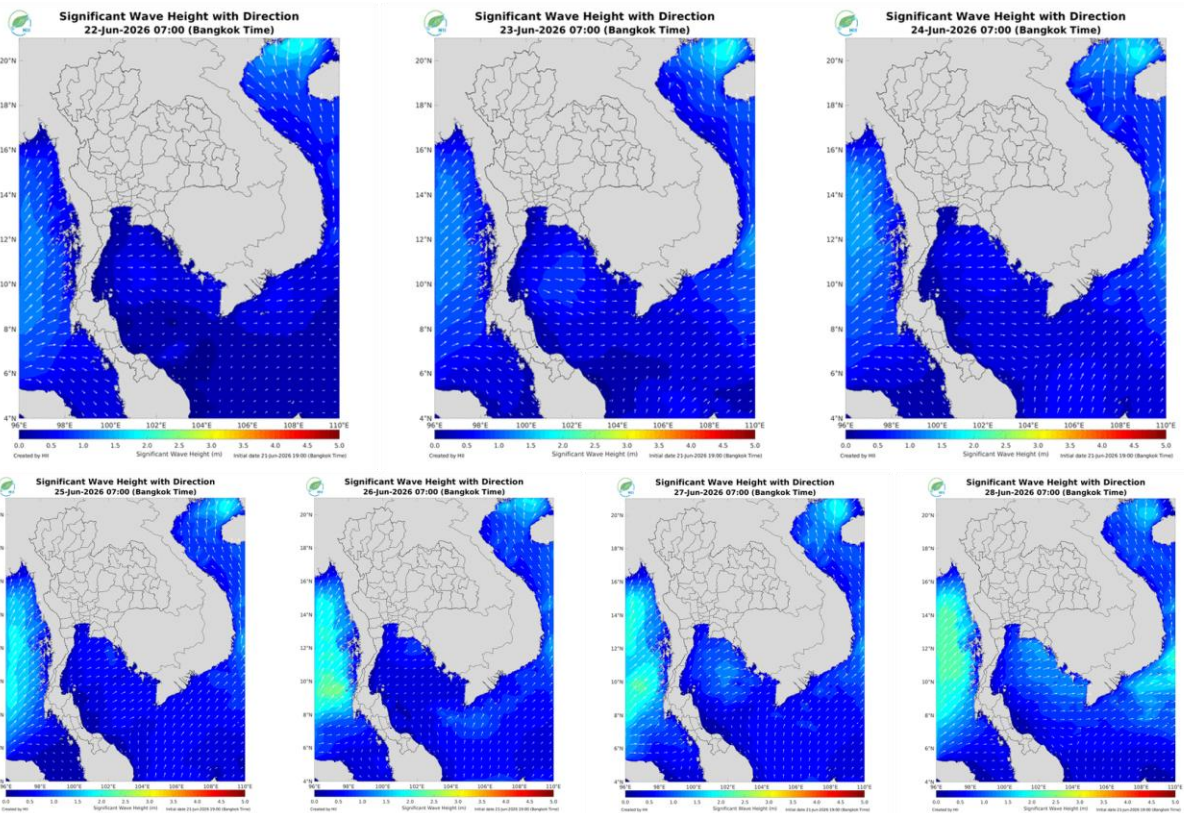
การคาดการณ์ความสูงและทิศทางคลื่นทะเล ระหว่างวันที่ 22 - 28 มิ.ย. 69
